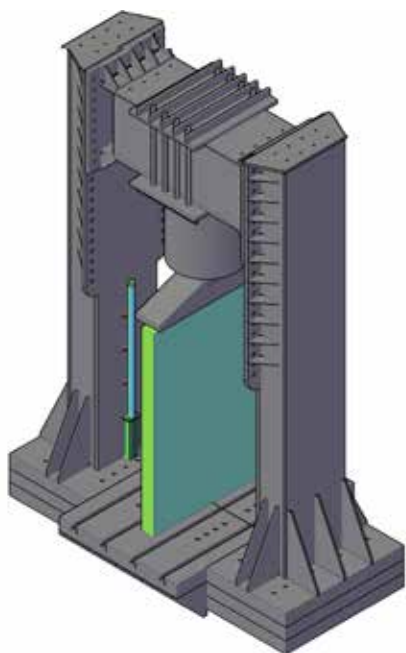
Стенд для испытаний крупногабаритных конструкций с нагрузкой до 15 000 кН
