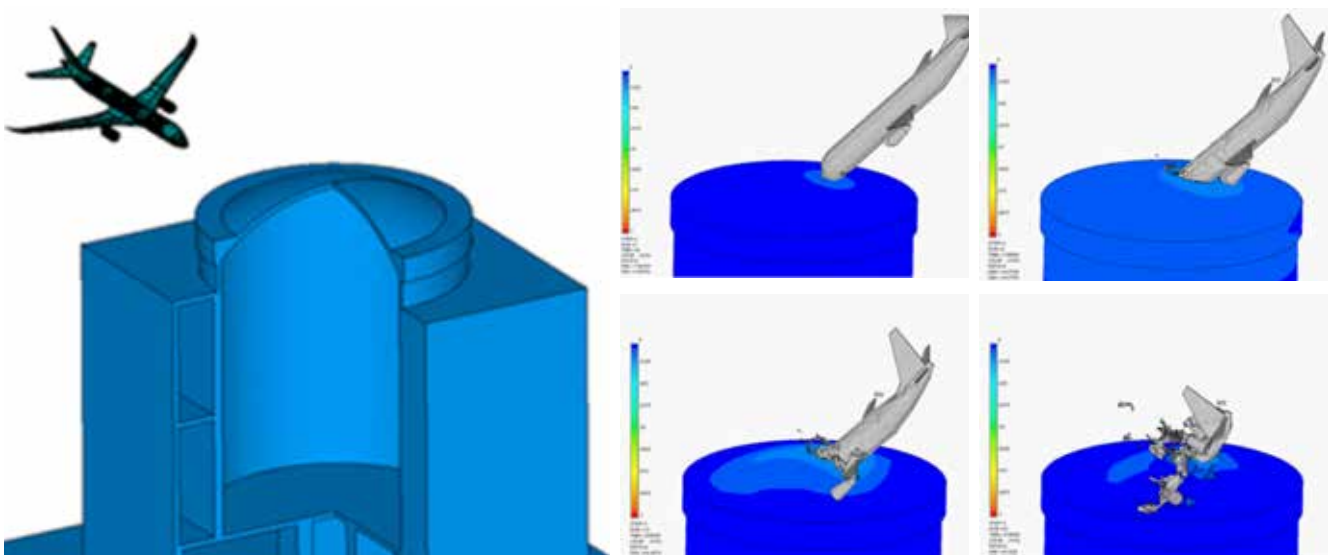
Разработка, программно-алгоритмическая реализация, верификация и апробация на объектах отрасли (проект ВВЭР-ТОИ) методик уточненного численного моделирования основных, особых и аварийных нагрузок и воздействий (ветровые и снеговые нагрузки, удар самолета, воздействия ударной волны, сейсмические воздействия, цунами, торнадо) на основные сооружения АЭС
