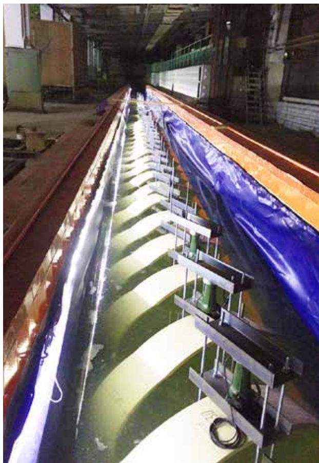
Проведение долгосрочных испытаний образцов стеклокомпозитных труб в соответствии с ГОСТ Р ИСО 10467-2013
