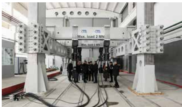
Универсальный реконфигурируемый стенд для испытаний крупногабаритных конструкций на статические и динамические нагрузки (5000 кН)
