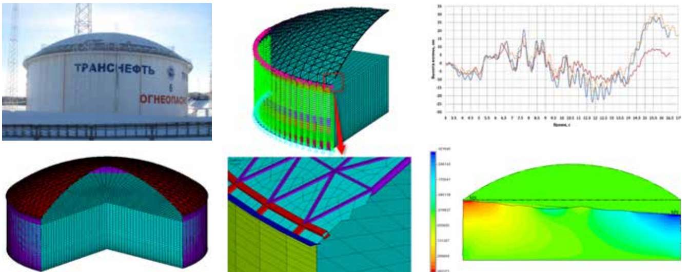
Резервуар РВСПА-50000 с нефтью в сейсмически активном районе. Решение связанных задач аэрогидроупругости
